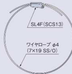
エンドレス仕様 組立例 (mm)
